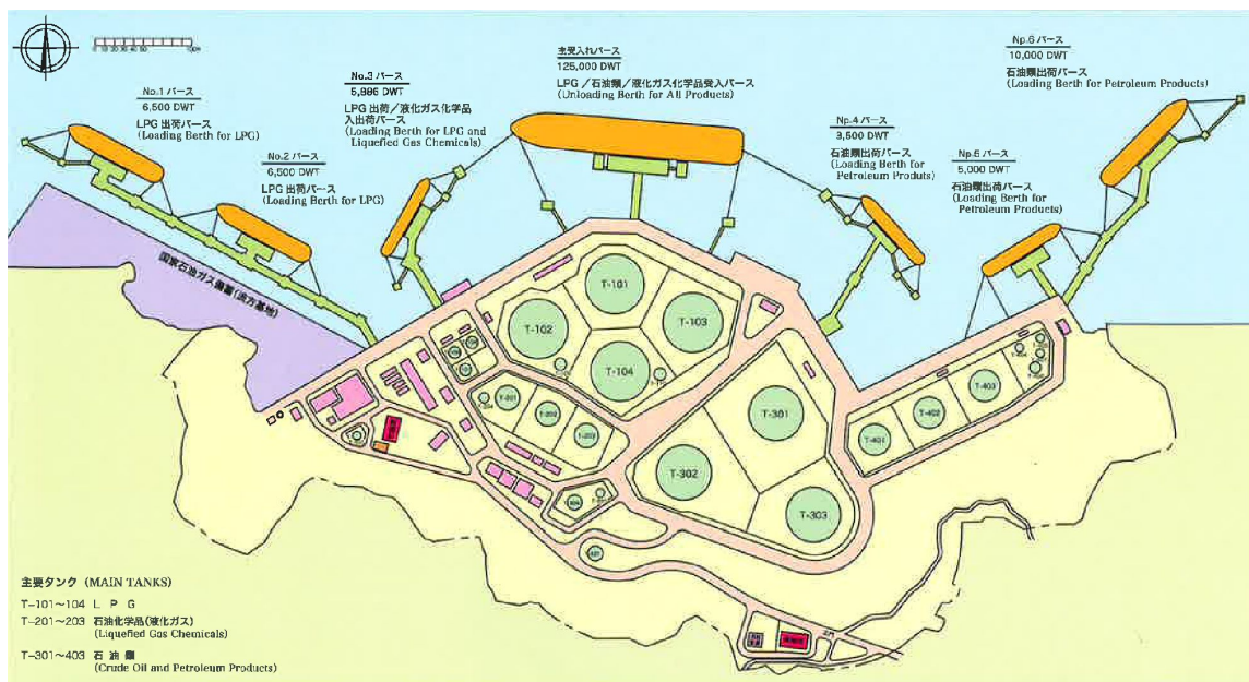
設備レイアウト図 出典：波方ターミナル株式会社案内パンフレット
