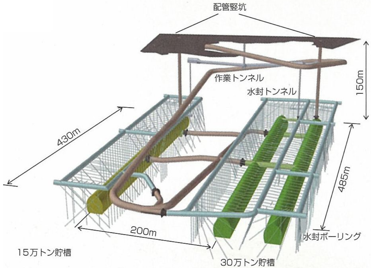
波方基地貯蔵施設概要図 出典：JOGMEC パンフレット「波方基地の概要」
