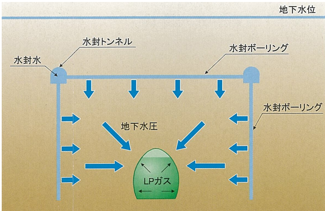
水封式地下岩盤貯蔵方式概念図 出典：JOGMEC パンフレット「波方基地の概要」
