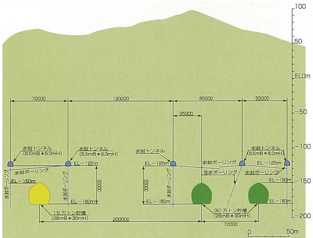
波方基地貯蔵施設断面図 出典：JOGMEC パンフレット「波方基地の概要」
